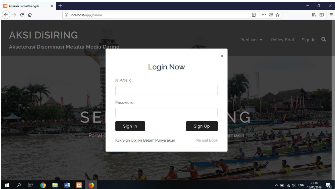
Gambar 3. Menu Login
