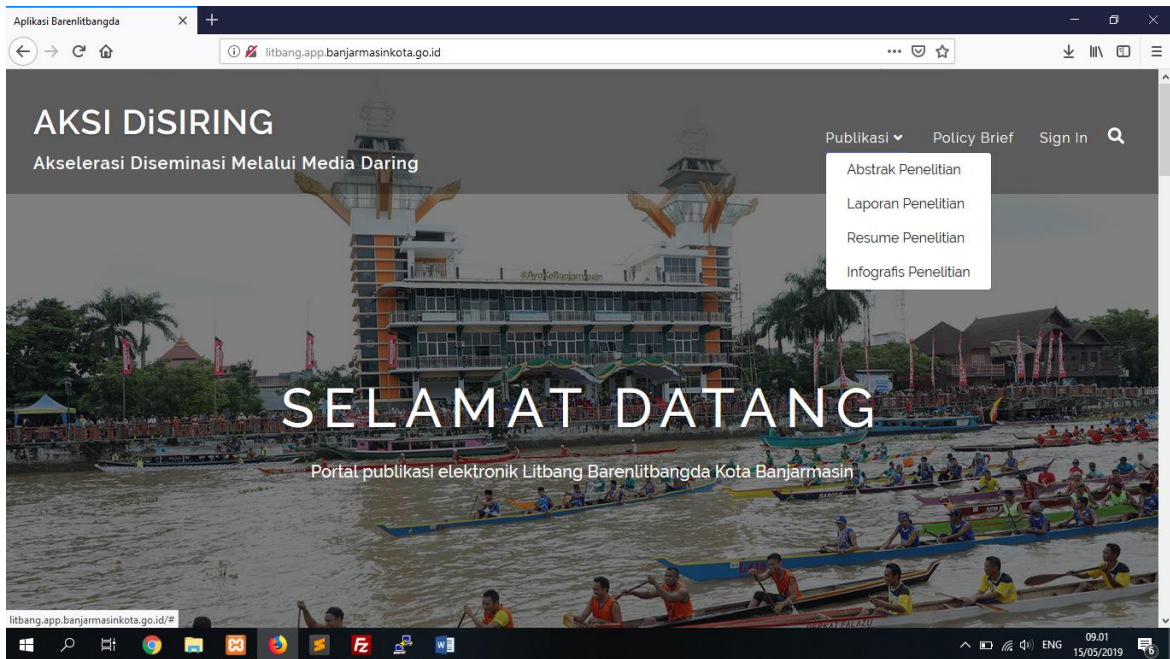
Gambar 2. Menu Laporan
